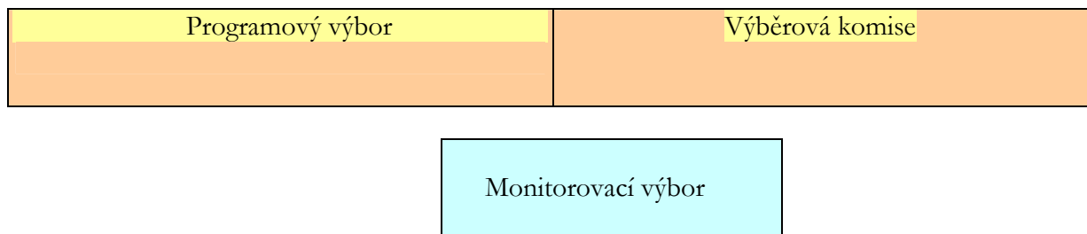
Obr. 4 Struktura MAS
